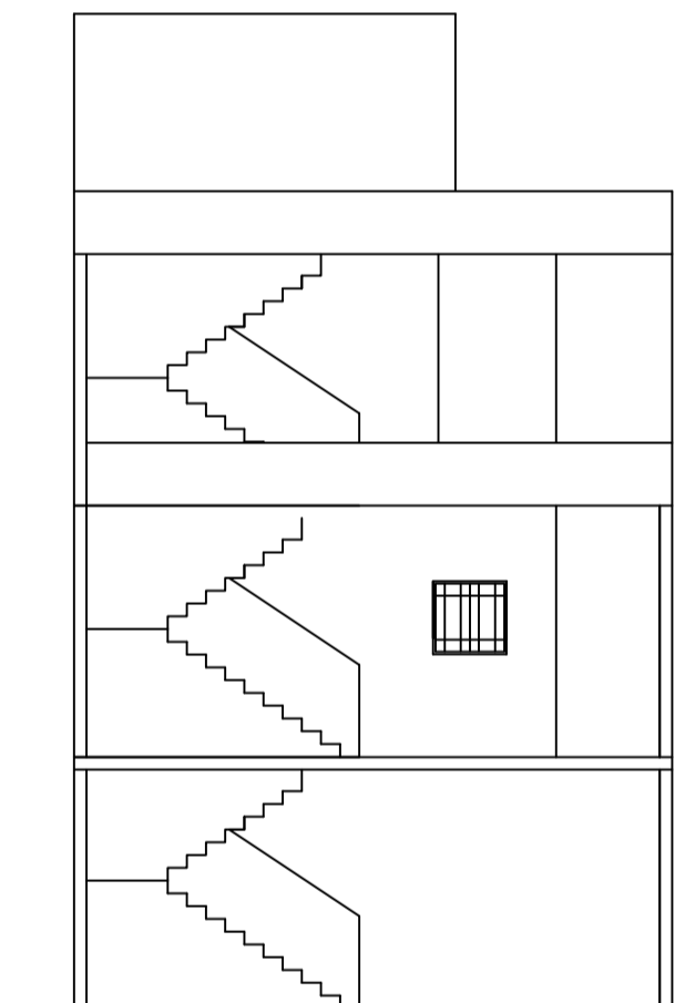
ELEVATION
